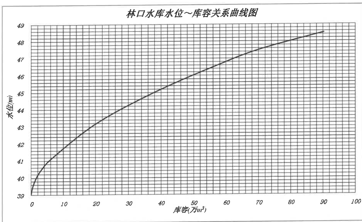
水位~库容关系曲线图
