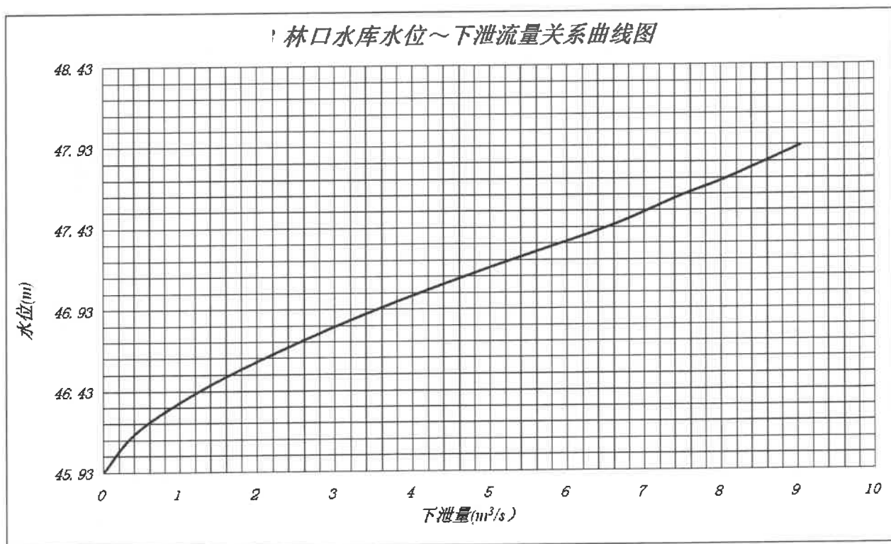
水位~下泄流量关系曲线图
